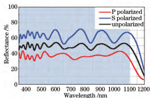
图 3 50:50 分束片的反射系数(350~1100 nm)
